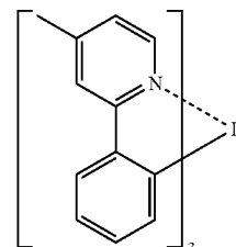
Ir(mppy) 3
