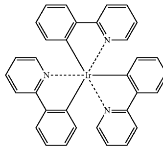
Ir(ppy) 3
