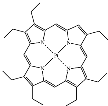
PtOEP
