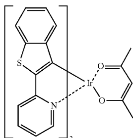
Btp 2 Ir(acac)
