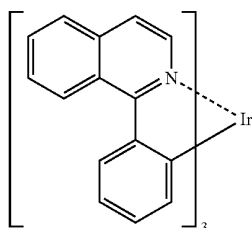
Ir(piq) 3
