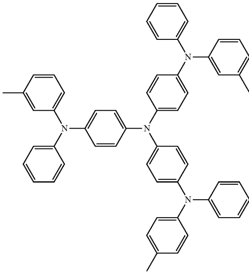
m-MTDATA
